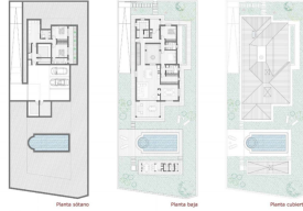
Planimetría
