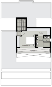
PLANTA ALTA
