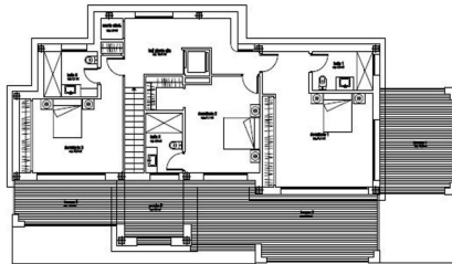
planta alta
