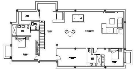
planta sótano
